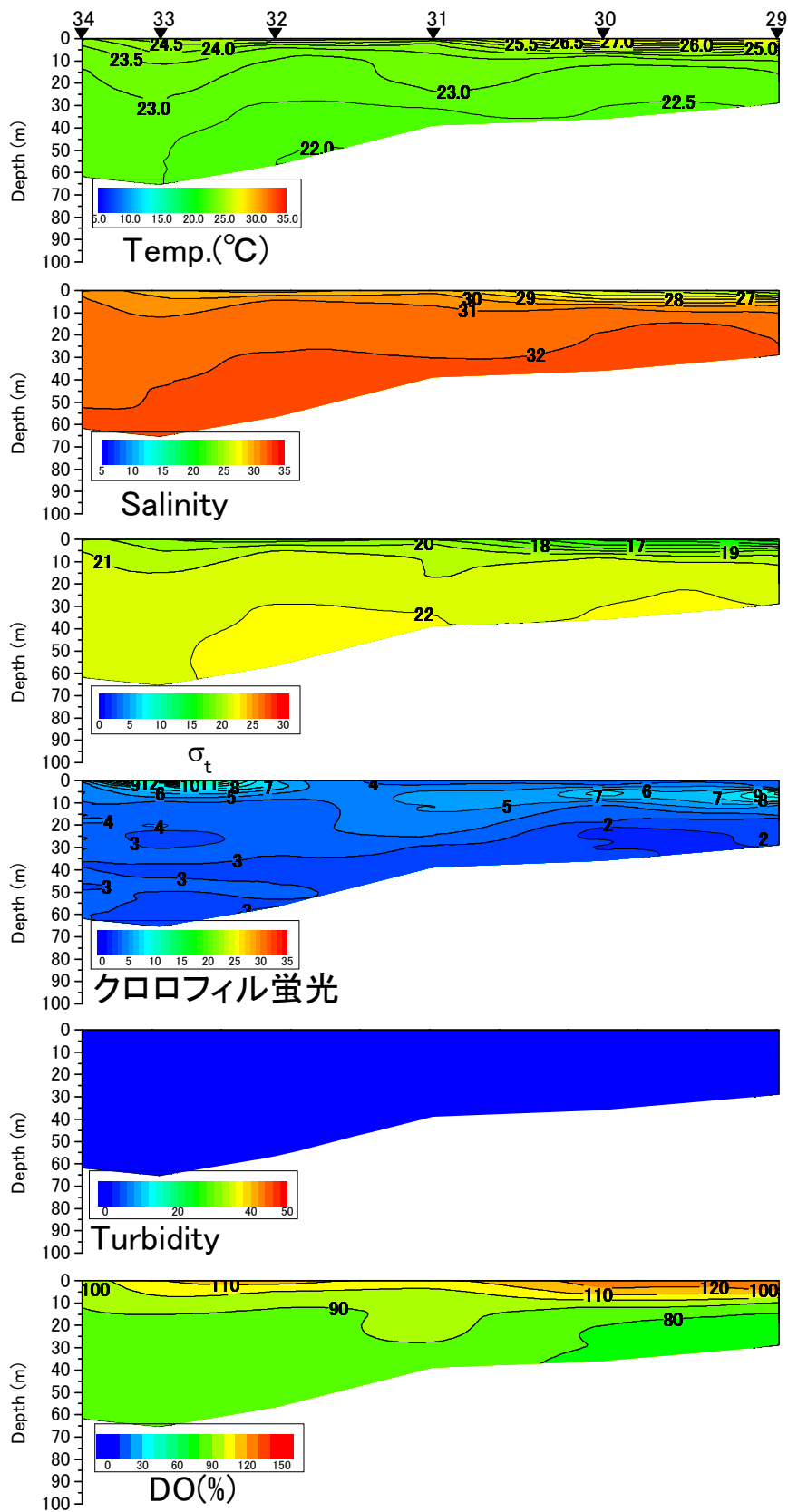
八代海西ラインの水温(°C)、塩分、密度( \sigma_t )、クロロフィル蛍光強度、濁度、溶存酸素飽和度(DO%)の鉛直面図(国土交通省の調査による) (2016年7月21日)
